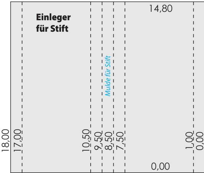
Faltansicht Einleger
